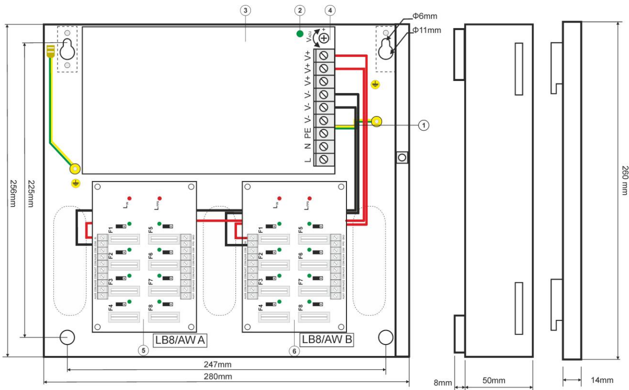
Rys.3. Widok zasilacza.
